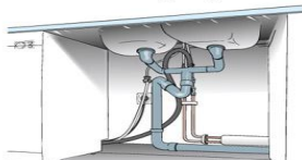
Rätt ansluten diskmaskin?
